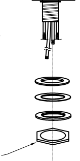
NUT
